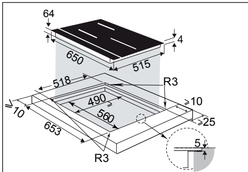
Bündiger Einbau
