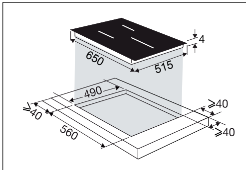
Einbau in eine Arbeitsplatte
