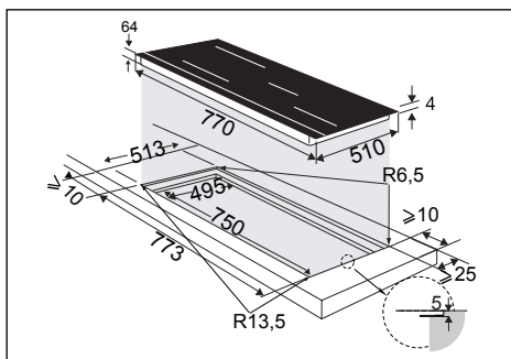
Inbouw in het werkblad
