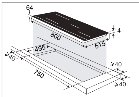
Osadenie do pracovnej dosky
