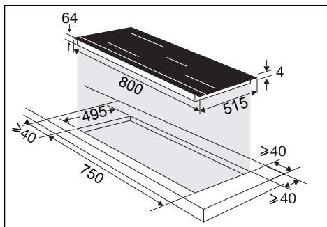
Inbouw op het werkblad
