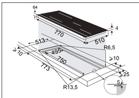
Osadenie na samotný povrch
